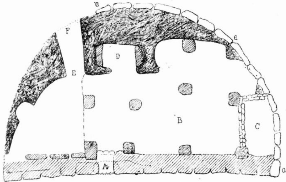
1. Plano de la sala hipóstila de Binigaus Nou (Migjorn Gran, Menorca), conocida por «Es Galliner de Madona», según E. Cartailhac, 1892.
