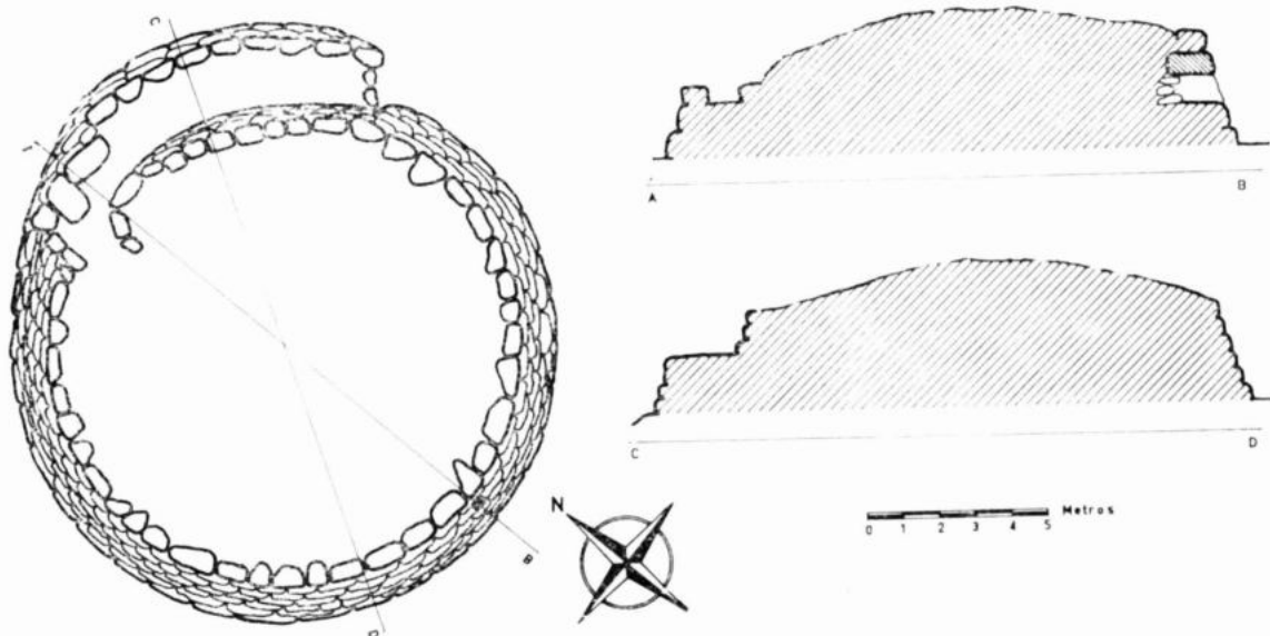
Fig. 4. — Biniatzén, Tanca de Sa Talaieta (Migjorn Gran). El portal que figura en corte A-B está basado en las medidas que da Chamberlin ( The Balearics , pág. 208), pues no fue posible dibujarlo directamente a causa de la tupida vegetación.
