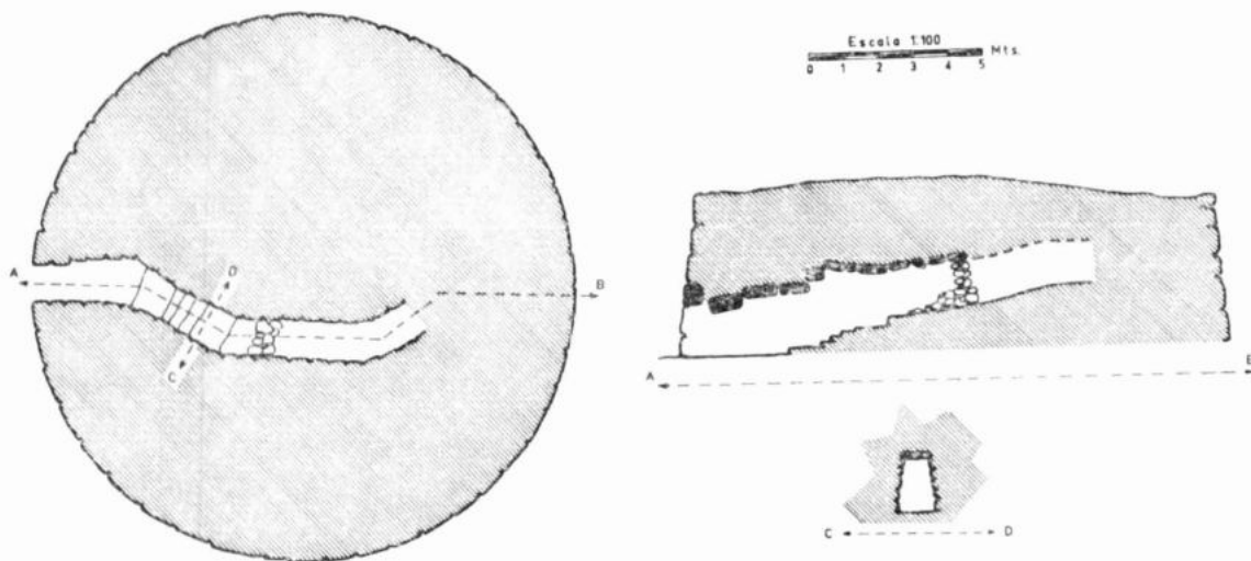
Fig. 3. — Tanca de Sa Talaia, Biniatzén (Migjorn Gran) (Mercadal). El diàmetre del monument es el que da Juan Hernández Mora en su Menorca Prehistòrica. Notes Descriptives , publicado en la Revista de Menorca , Mahón, 1948, pág. 264, pues actualmente el estado ruinoso de algunas partes del talaiot y la tupida vegetación que lo recubre impiden medirlo.
