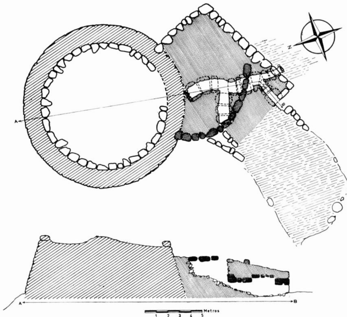
Fig. 7. — Santa Mònica (Migjorn Gran) (Mercadal).
